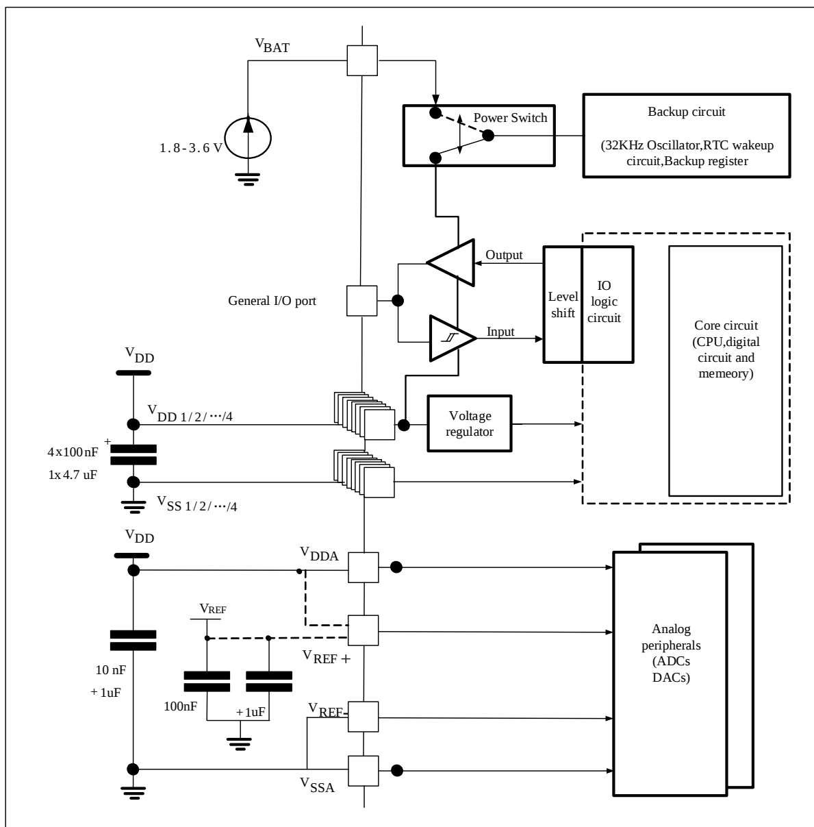
图 4-3 供电方案
