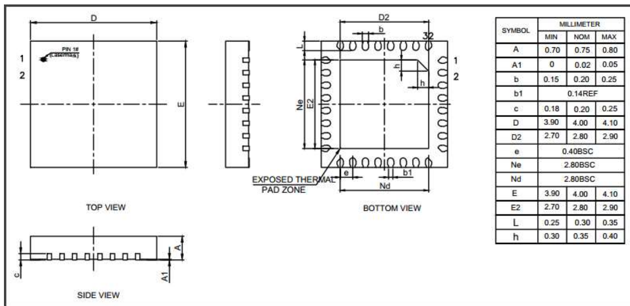
图 5-1 QFN32封装尺寸
